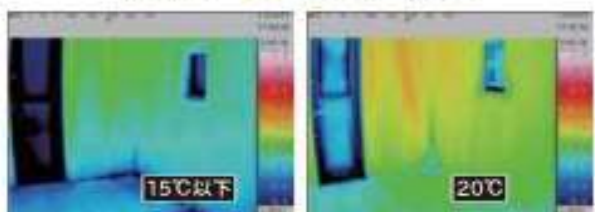
一般の断熱工法 アクアフォーム®と断熱サッシ
